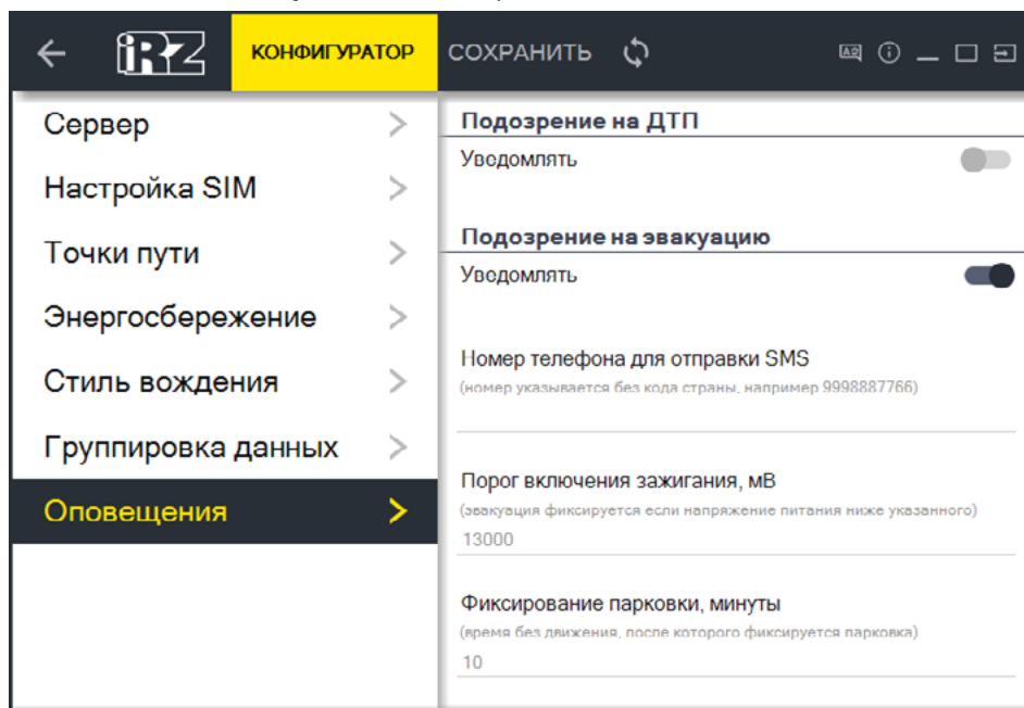
Рис. 3.8. Вкладка «Оповещения»
